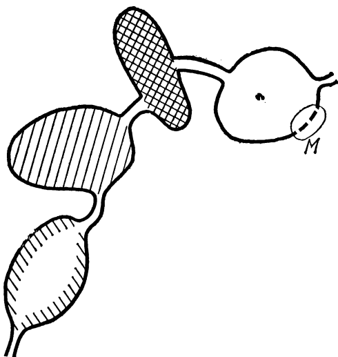
Рис. 3. «Вечная» Вселенная. Каждый «овал» представляет мини-вселенную со своим набором фундаментальных констант, которая в процессе эволюции порождает новую мини-вселенную, и так до бесконечности. На рисунке изображены топологически связанные мини-вселенные. Однако сейчас нельзя исключить, что Вселенная состоит из топологически несвязанных областей. Буквой M символически помечена наша Метагалактика, являющаяся весьма малой частью одной мини-вселенной
