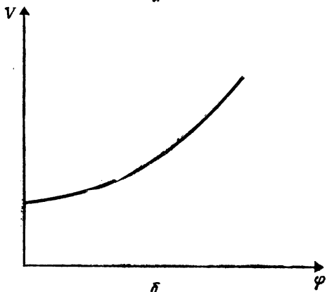
Рис. 2. а) Плотность энергии V(\varphi) при T \rightarrow 0 в модели хаотической Вселенной. Флуктуирующее возмущение (шарик) проходит через потенциальный барьер; в это время осуществляется «раздувание»; б) зависимость плотности потенциальной энергии V(\varphi) при T \rightarrow \infty
