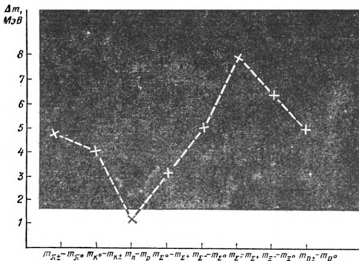
Рис. 5. Распределение изотопических семейств по разностям масс. По оси абсцисс указаны разности масс для соответствующего изотопического семейства, по оси ординат — величина этой разности, выраженная в энергетических единицах
